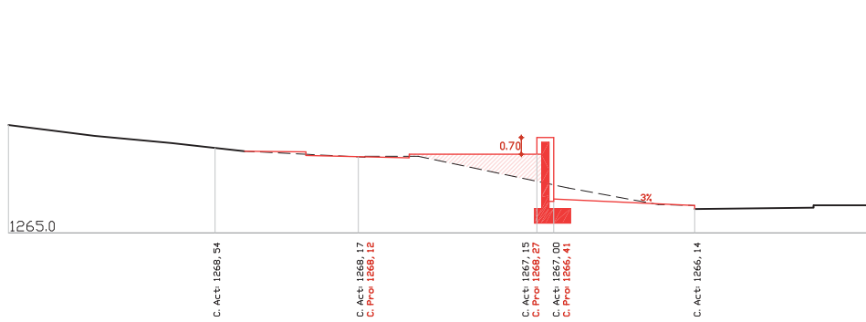
SECCIÓ LONGITUDINAL (1)
