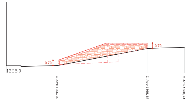
SECCIÓ LONGITUDINAL (2)
